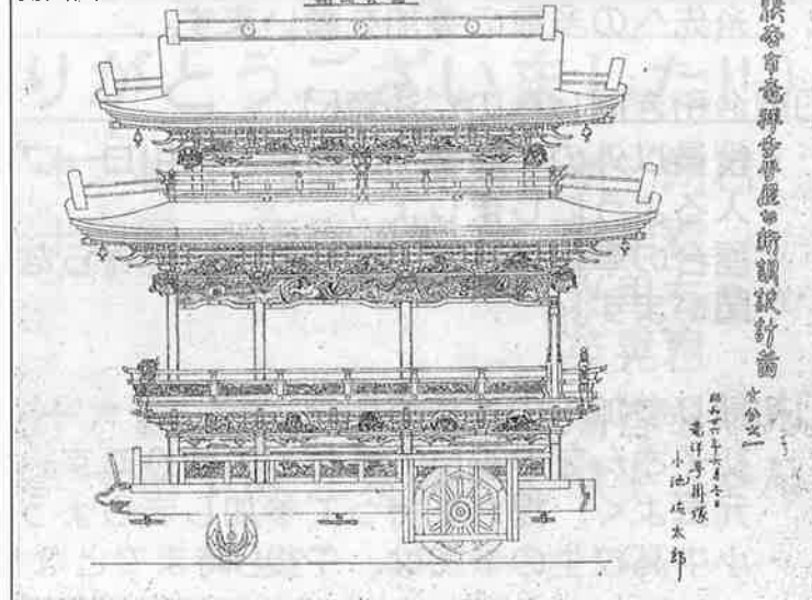
側面図
